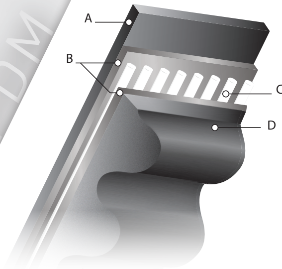
A : protection haute résistance B : mélange de liaison spécifique EPDM C : câblé haute résistance, faible allongement (polyester renforcé raidi) D : mélange EPDM renforcé avec fibres orientées
